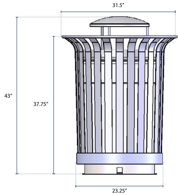
RB Dimensions
